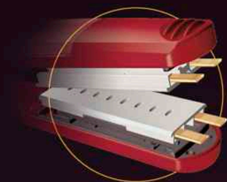
4 elementos térmicos em cerâmica 4 ceramic heating elements
